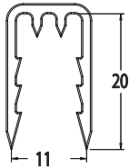
450-8211 11x20x20 Grip 2mm wire
