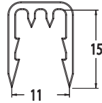
440-8111 11x15x15 Grip 1.5mm wire
