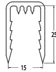
470-8115 15x25x25 Grip 3mm wire
