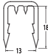
450-8113 13x18x18 Grip 2mm wire
