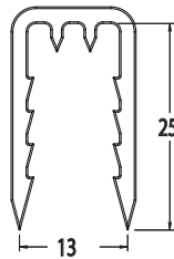
470-8113 13x25x25 Grip 3mm wire
